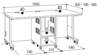
▲CAI-16X1W寸法図
