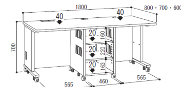
▲CAI-18X1W寸法図
